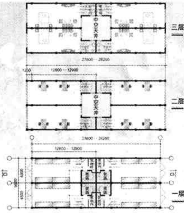
P型II(铝)四P组合平面图 P建筑面积约168m²
